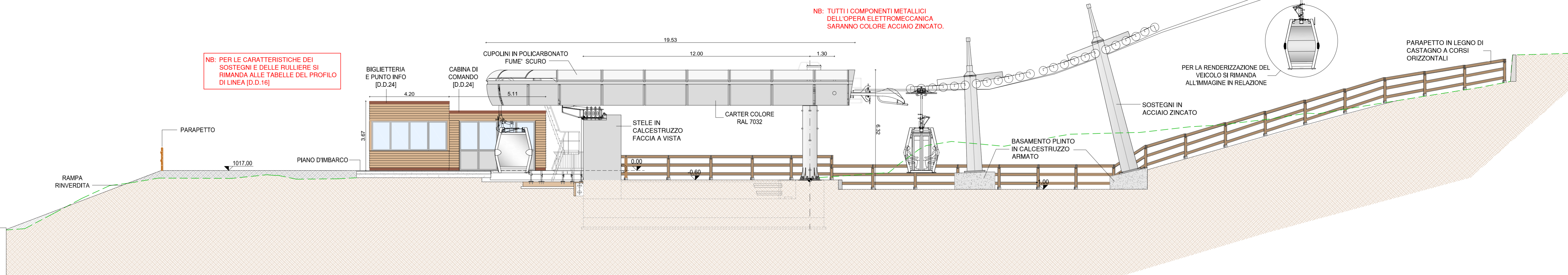
PROSPETTO LONGITUDINALE STAZIONE DI VALLE
